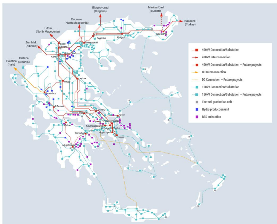
希腊电网分布图
