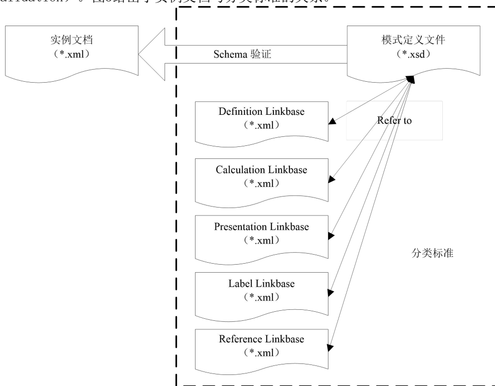
图3 实例文档与分类标准的关系
