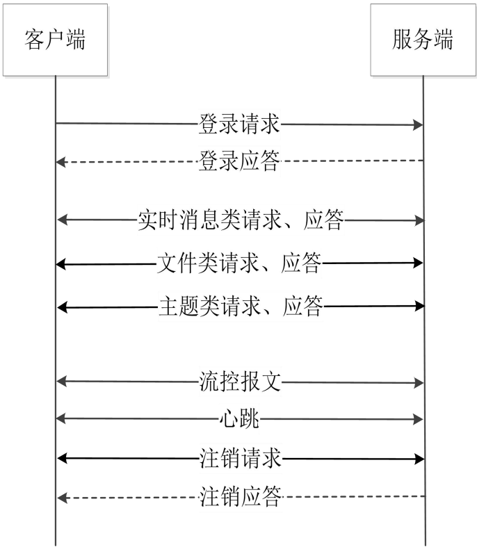
图 5 会话流程图
