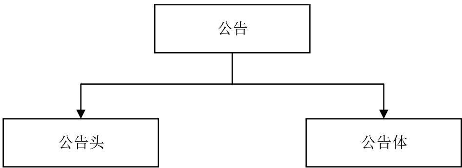
图 1 公告的结构
